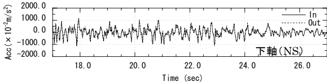
(a) 加速度波形 (10Hzのハイカットフィルター)
