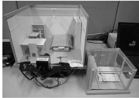
写真 4 室内模型 (左: 1/10 洋室, 右: 1/20 和室)
