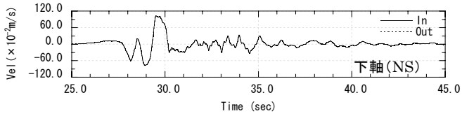
(a)速度波形 (10Hzのハイカットフィルター)
