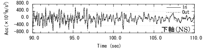
(a) 加速度波形 (10Hzのハイカットフィルター)
