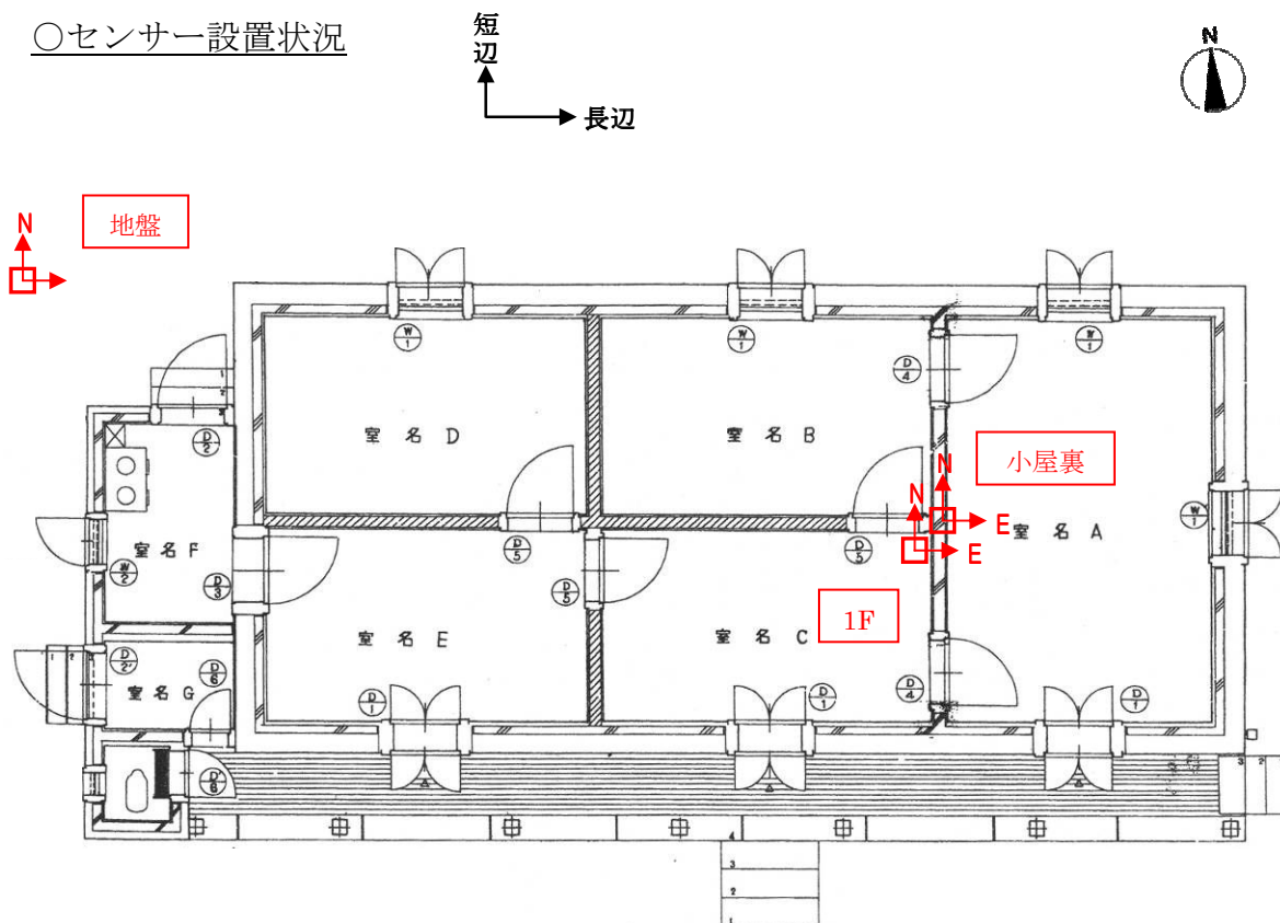
1 階平面図
