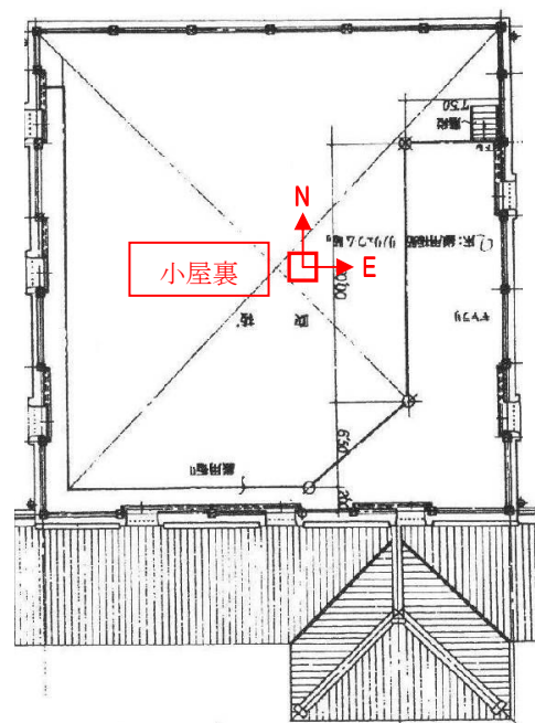
2 階平面図
