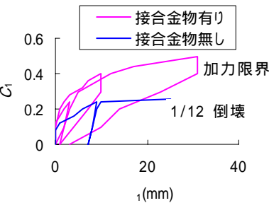
図1 1階の復元力特性
