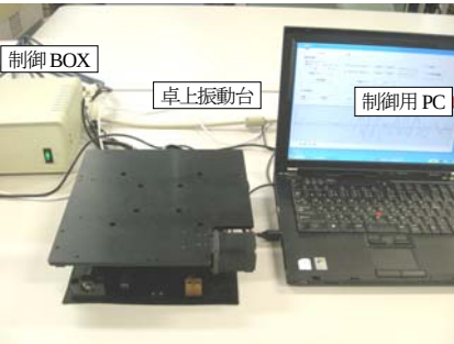
図 1 卓上振動台の構成と形状
