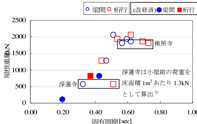
図 4 固有周期と屋根荷重の関係
