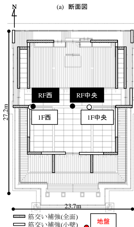
(b) 平面図 図 2 浄蓮寺
