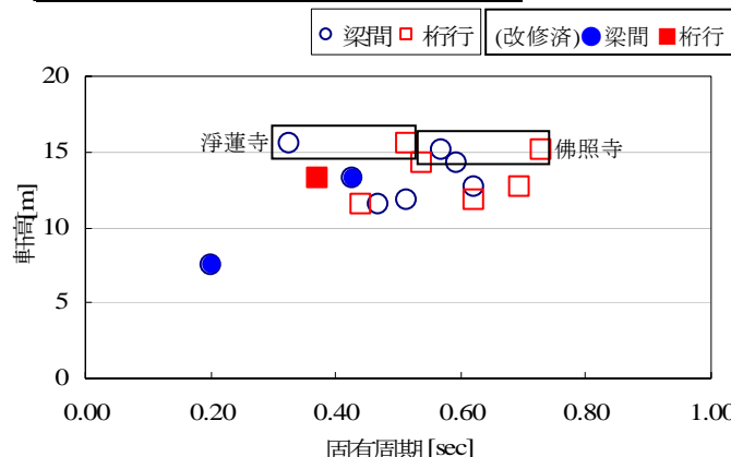
図 3 固有周期と軒高の関係
