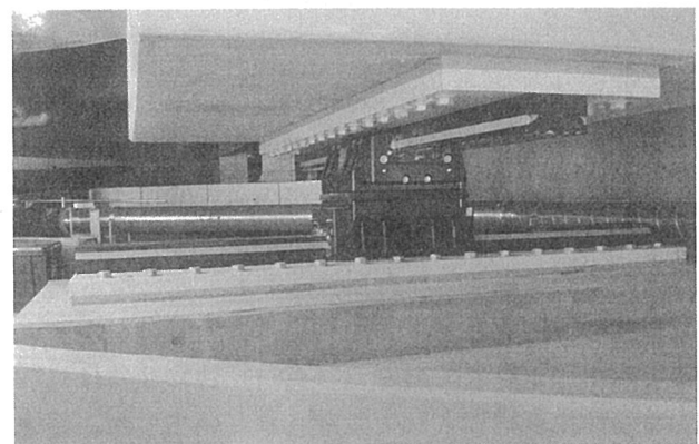
写真7 免震装置 (直動転がり支承)
