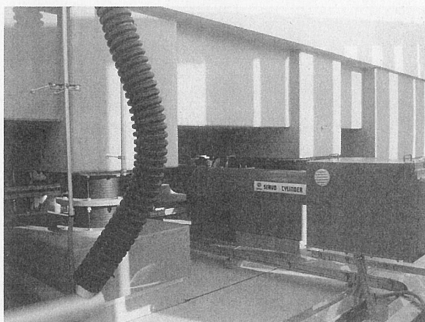
写真8 屋上実験室 免震装置 (アクチュエータ、積層ゴム支承)
