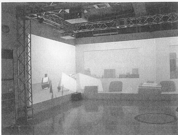
写真9 屋上実験室内 地震時家具挙動の動画
