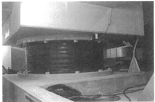
写真6 免震装置 (積層ゴム支承)
