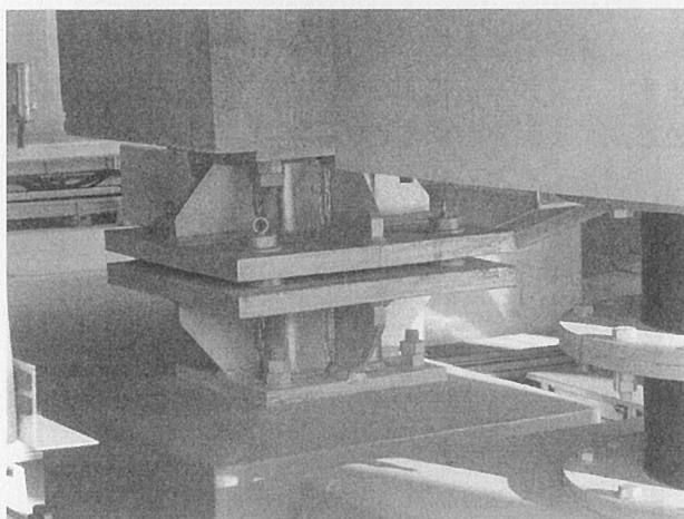
写真11 屋上実験室下免震層 シアピン
