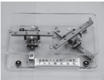
写真5 免震層部品
