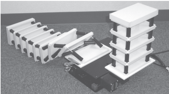
写真3 8階建て模型の倒壊
