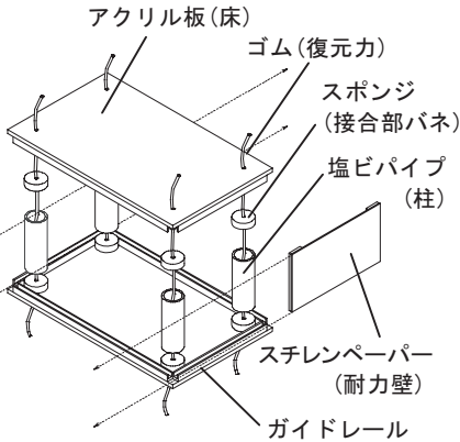
図1 建物模型の詳細
