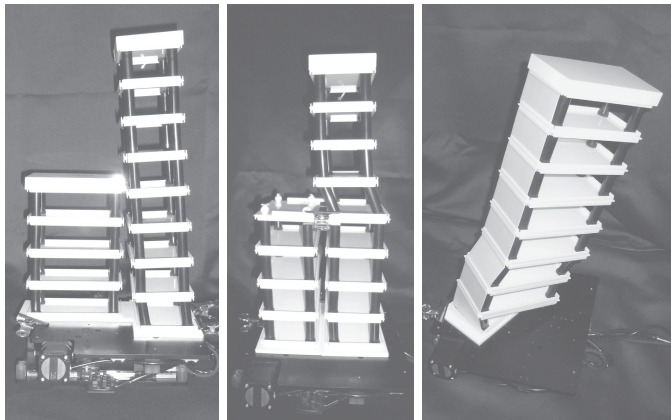
(a) 頂部の衝突 (b) 剛性率の変化 (c) 偏心による振れ
